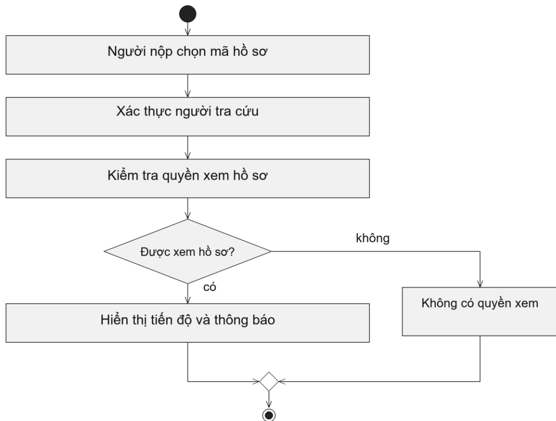
Biểu đồ hoạt động UC08 Theo dõi tiến trình hồ sơ
