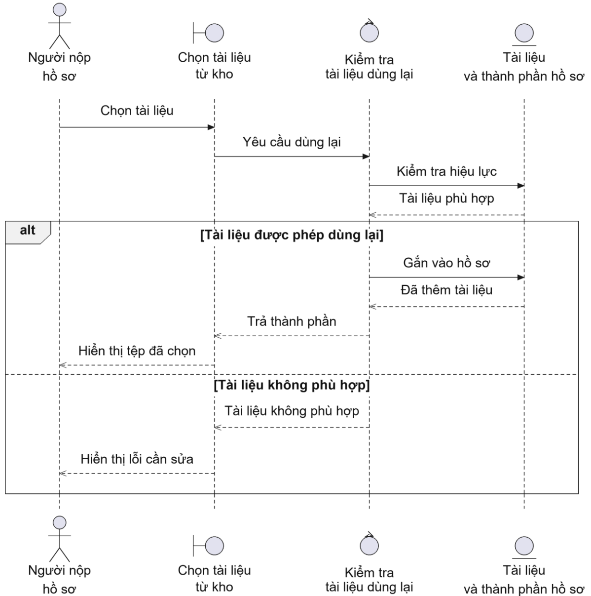
Hình 2.110: Biểu đồ trình tự của Use case UC29
